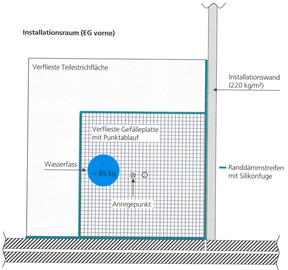
Lage des Prüfaufbaus im Installationsraum (EG vorne).
