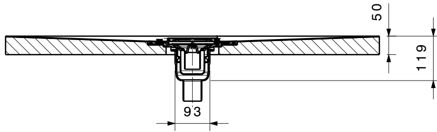
Schnittansicht A-A (2)
