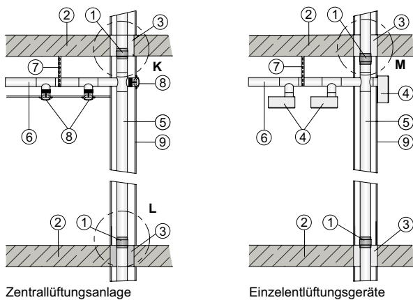
Zentrallüftungsanlage
