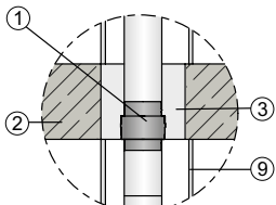
Einbau in Geschosdecke aus Beton
