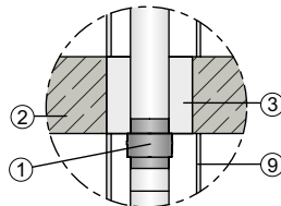
Einbau unter der Geschosdecke aus Beton. Befestigung über 3 mm große, umlaufende Sicke.
