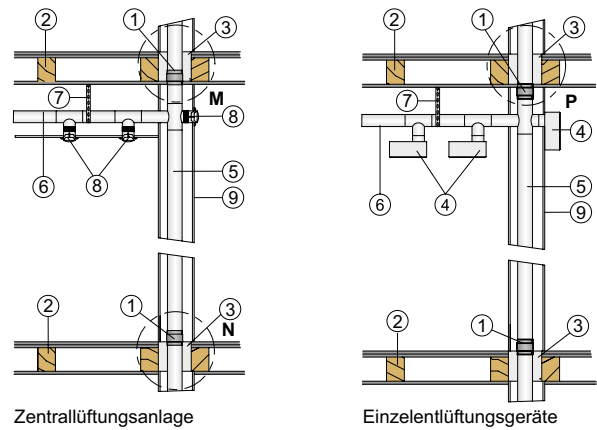
Zentrallüftungsanlage
