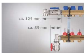
Verteiler-Anschluss-Set 90° (Art.-Nr. 291100)
