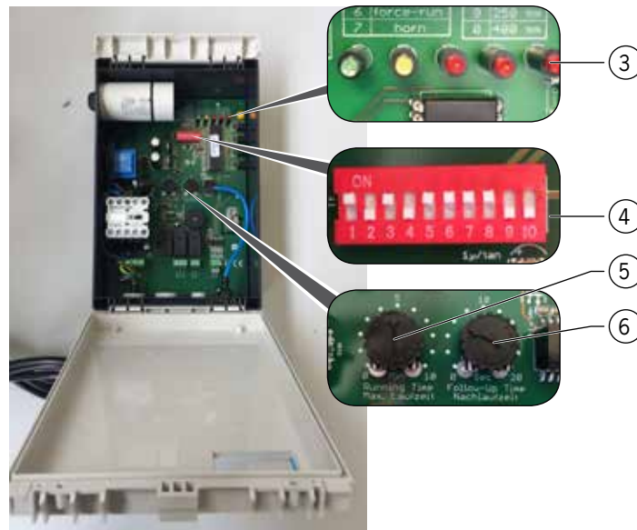
Abbildung: Übersicht der Bedien- und Anzeigenelemente –Innen –
