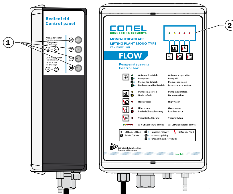
Abbildung: Übersicht der Bedien- und Anzeigenelemente –Außen –
