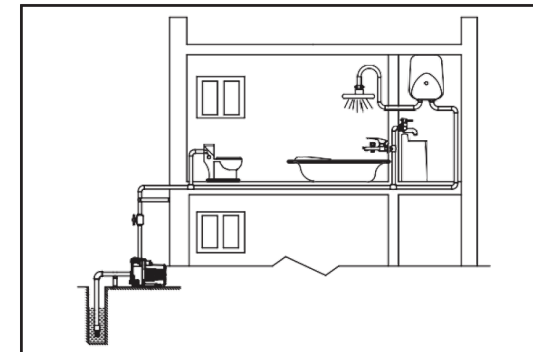
Abb. 10 Grundwasser für den Druckaufbau
