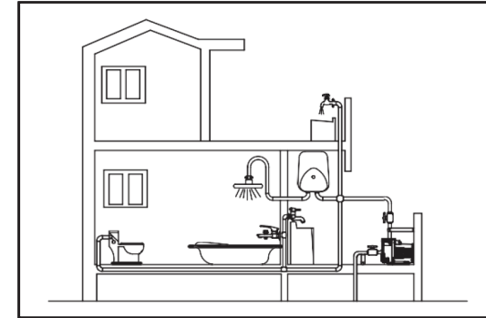
Abb. 9 Direktdruck Leitungswasser
