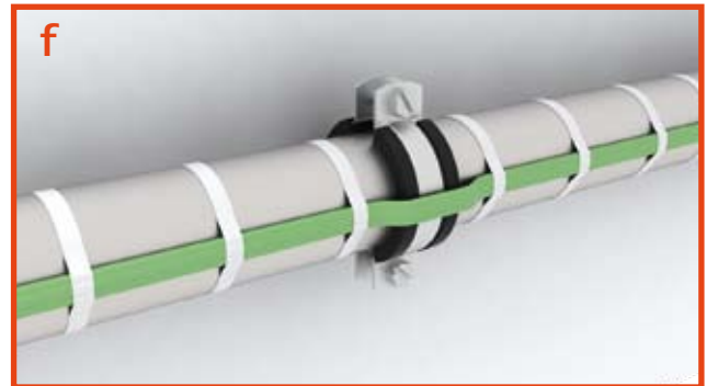
Verlegung an Schellen
